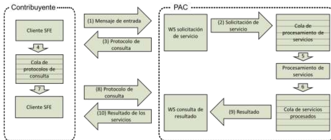
Ilustración 6 – Servicio Web Asincrónico
